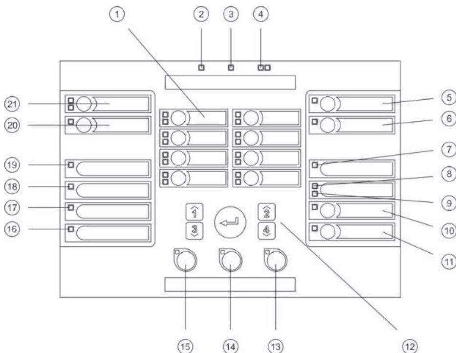
Bild 2: Användargränssnitt för åttasektioners centralapparater
