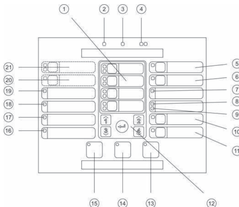
Obrázek 1: Uživatelské rozhraní pro dvou- a čtyřzónové ústředny
