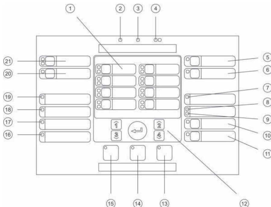
Figura 2: Interfaccia utente delle centrali a otto zone
