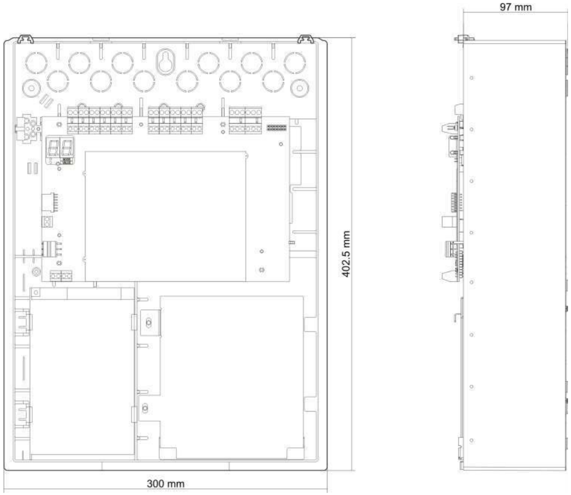
Şekil 22: İki ve dört bölümlü kapaksız kasa
