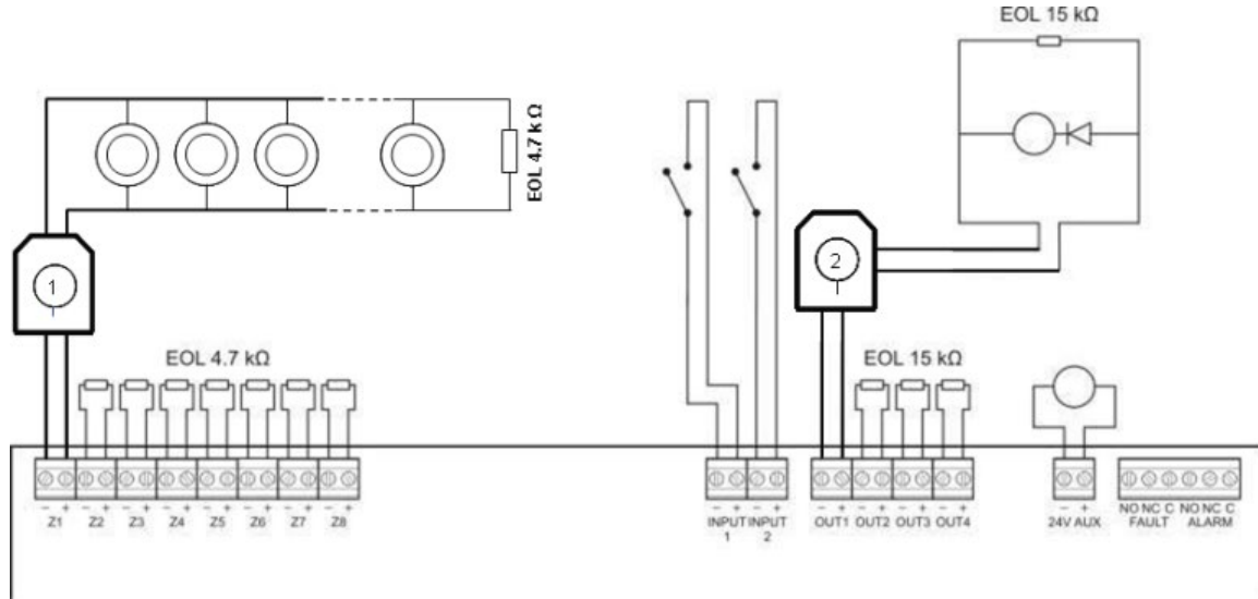
Şekil 7: Kendinden güvenli yangın sistemi bağlantıları
