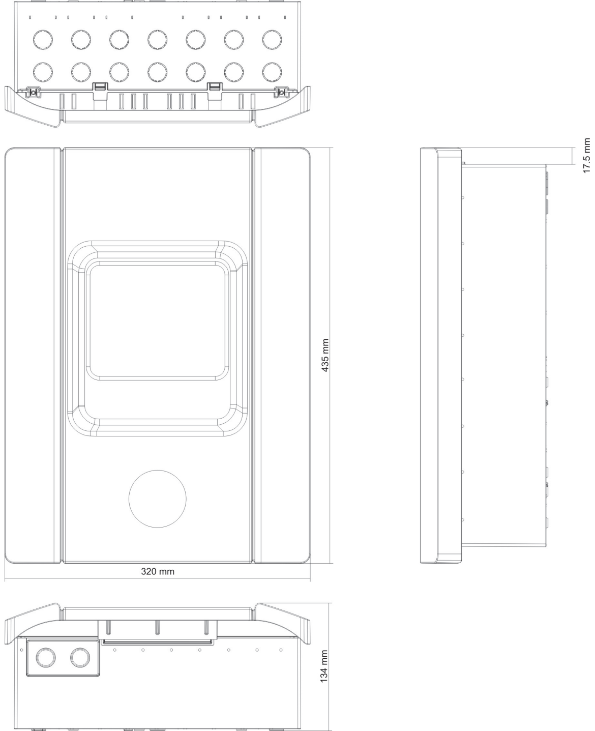
Şekil 21: İki ve dört bölge kapaklı kasa
