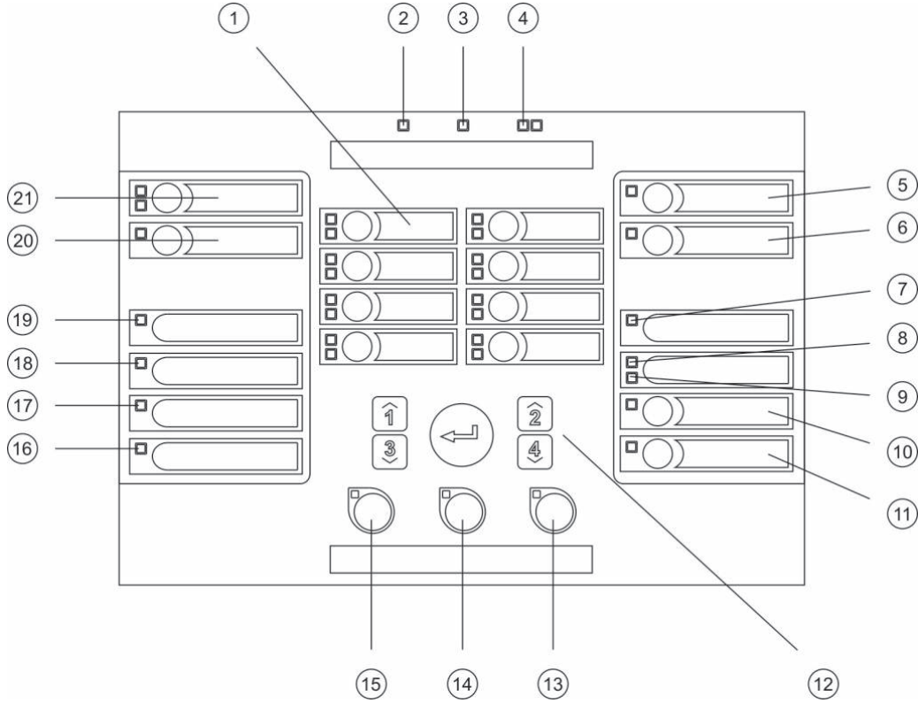
Şekil 17: Sekiz bölge kontrol panelleri için kullanıcı arayüzü
