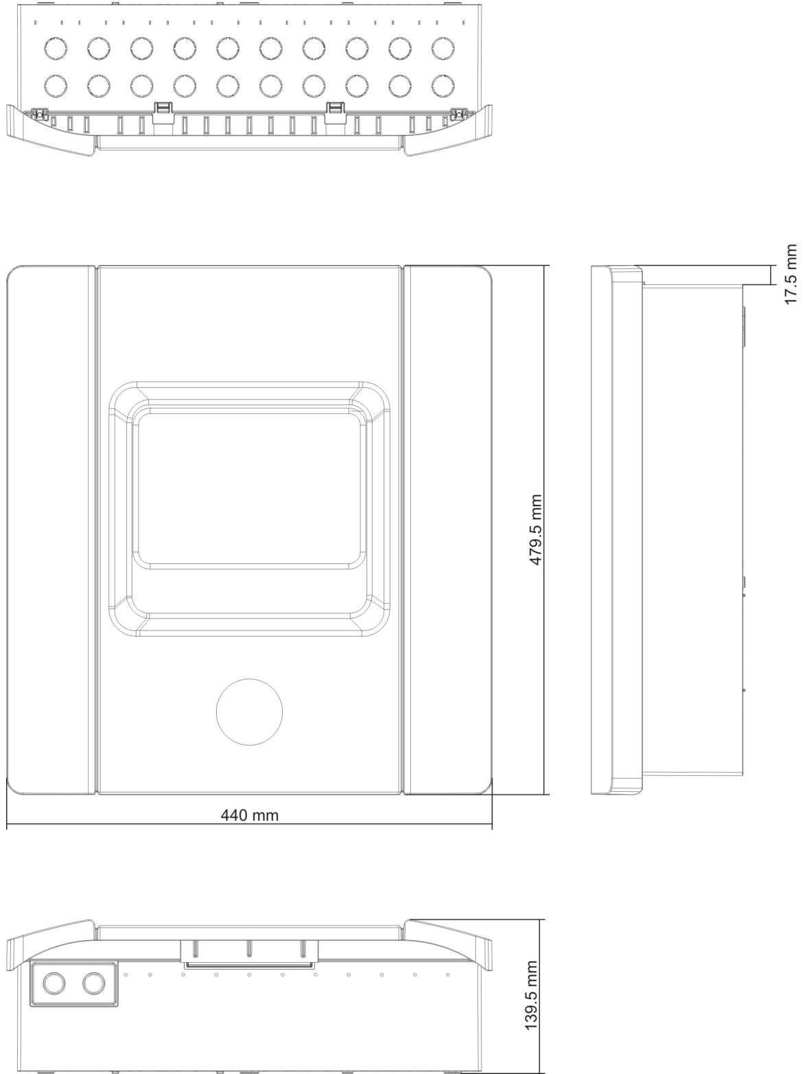
Şekil 23: Sekiz bölge kapaklı kasa
