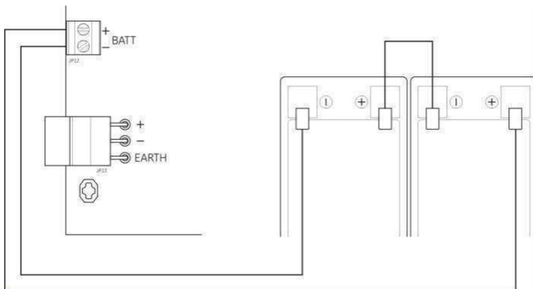
Afbeelding 12: Accu's aansluiten
