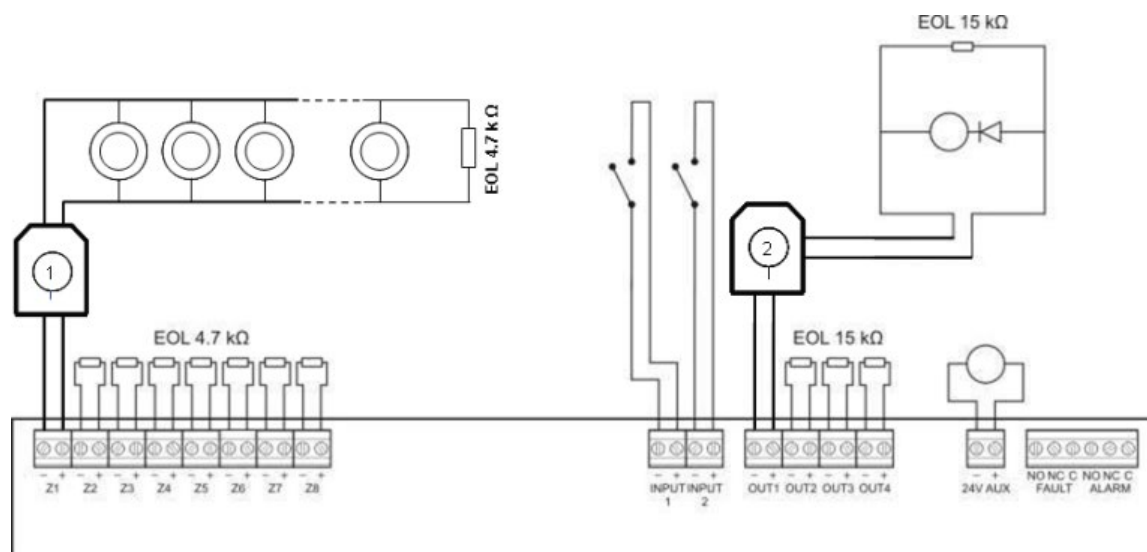
Afbeelding 7: Intrinsiek veilige aansluitingen van het brandmeldsysteem
