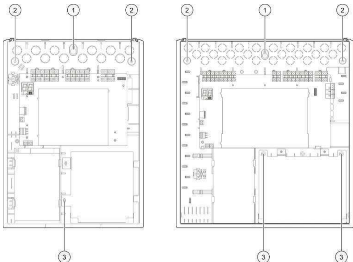
Afbeelding 3: Posities van de montagegaten
