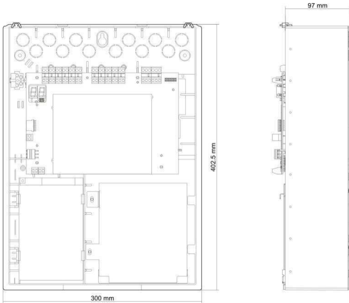
Abbeelding 22: Behuizing voor twee en vier groepen zonder deksel
