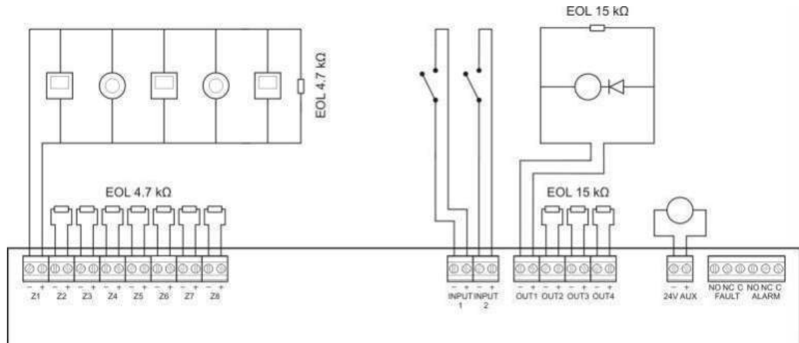
Afbeelding 4: Standaardaansluitingen van het brandmeldsysteem (geen EN 54-13-norm)
