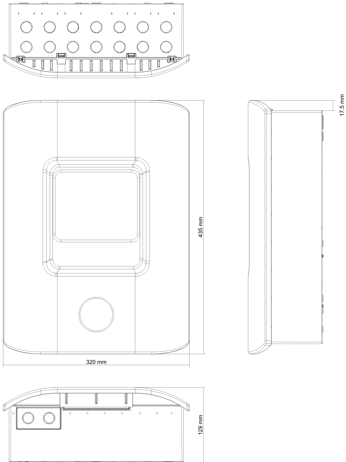
Figura 21: Dulap pentru panou cu două și patru zone cu capac
