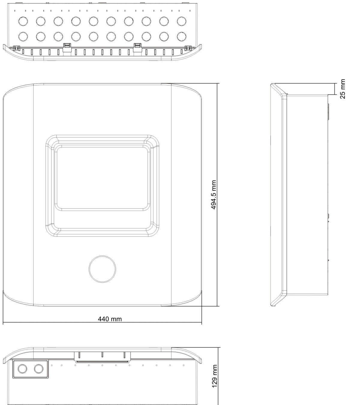
Figura 23: Dulap pentru panou cu opt zone cu capac
