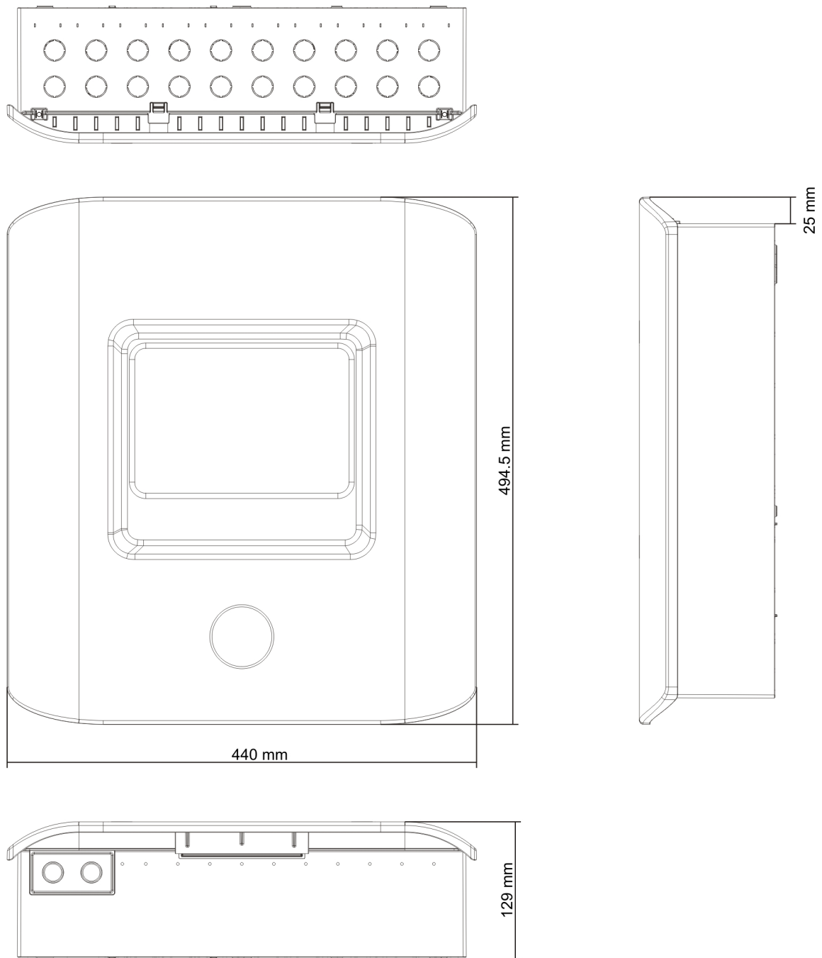
Figure 23 : Armoire à huit zones avec couvercle
