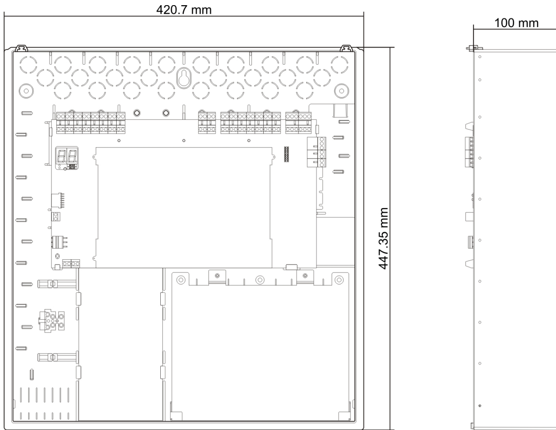
Figure 24 : Armoire à huit zones sans couvercle
