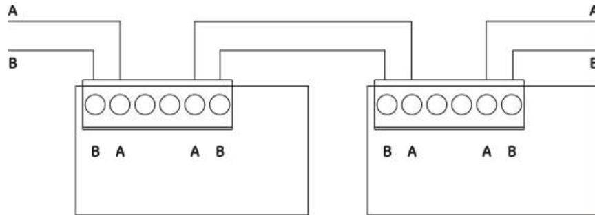
Figure 13 : Raccordements d'une carte réseau
