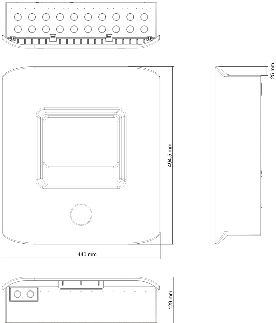
Bild 23: Åttasektioners skåp med hölje
