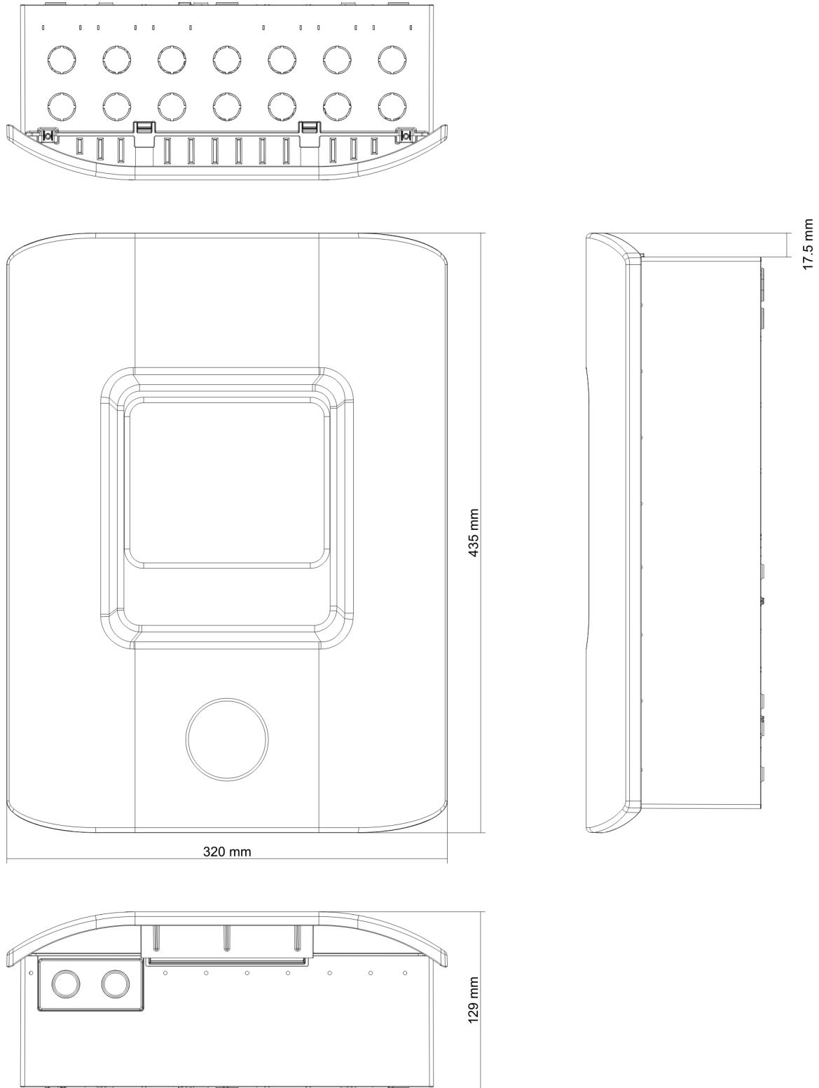
Bild 21: Två- och fyrasektioners skåp med hölje
