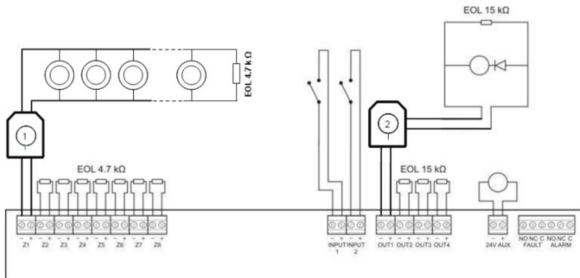
Bild 7: Egensäkra brandsystemanslutningar
