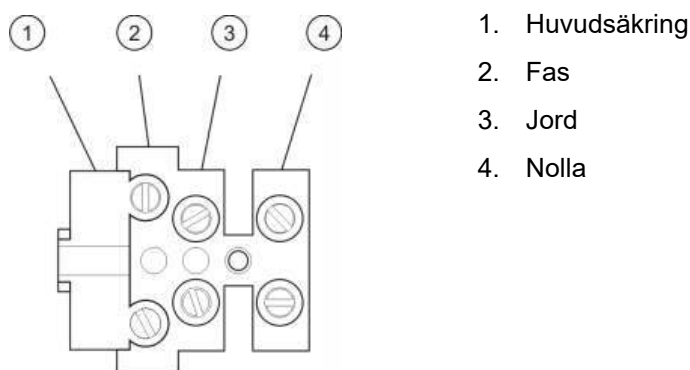
Bild 10: Ansluta nätspänning
