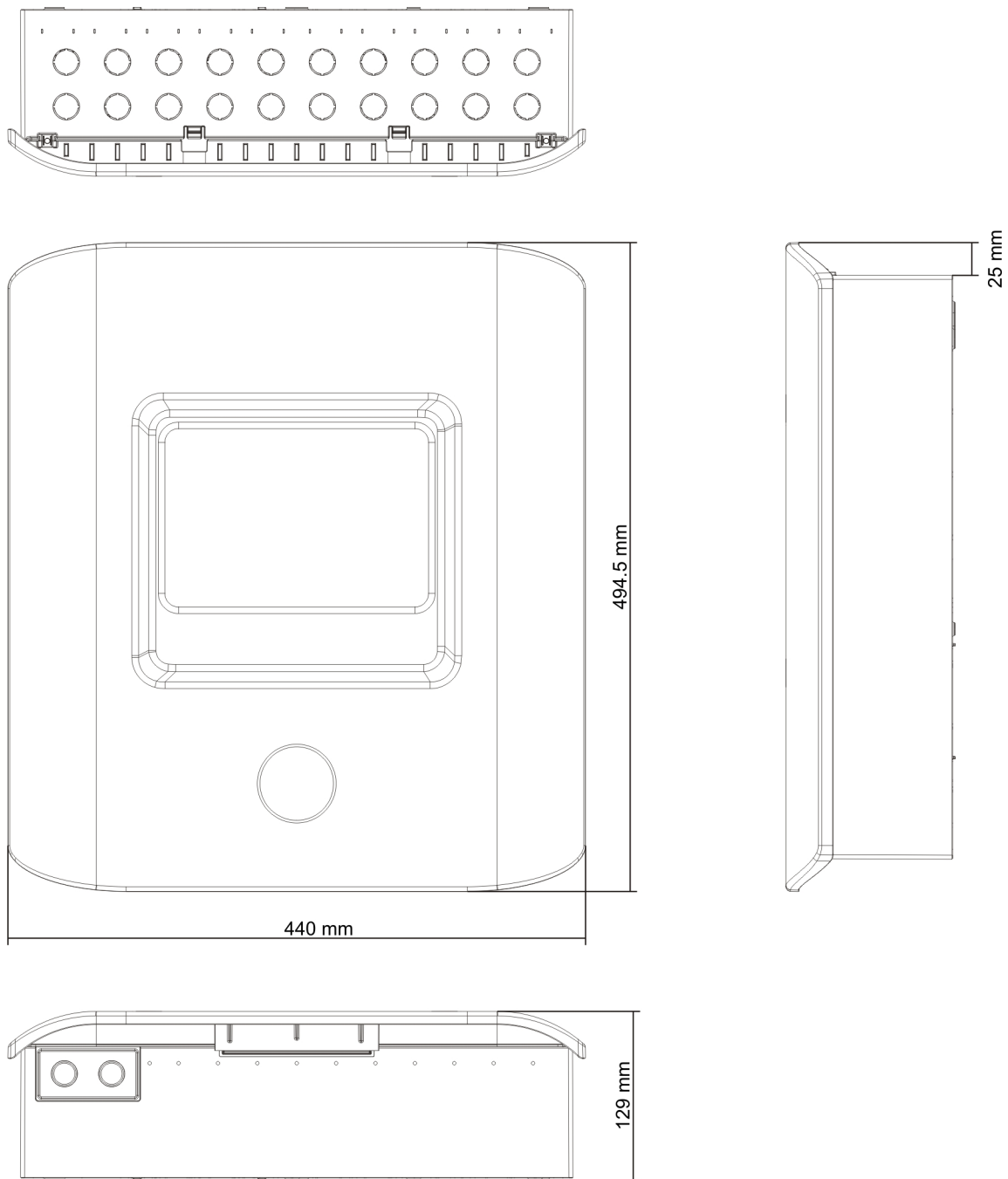
Afbeelding 23: Behuizing voor acht groepen met deksel
