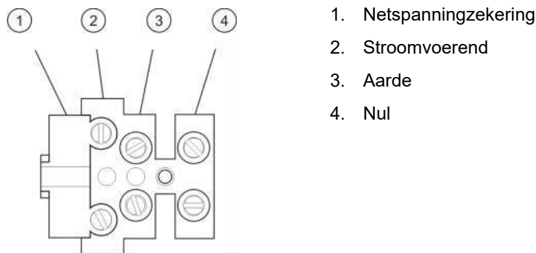
Afbeelding 10: Voedingseenheid aansluiten
