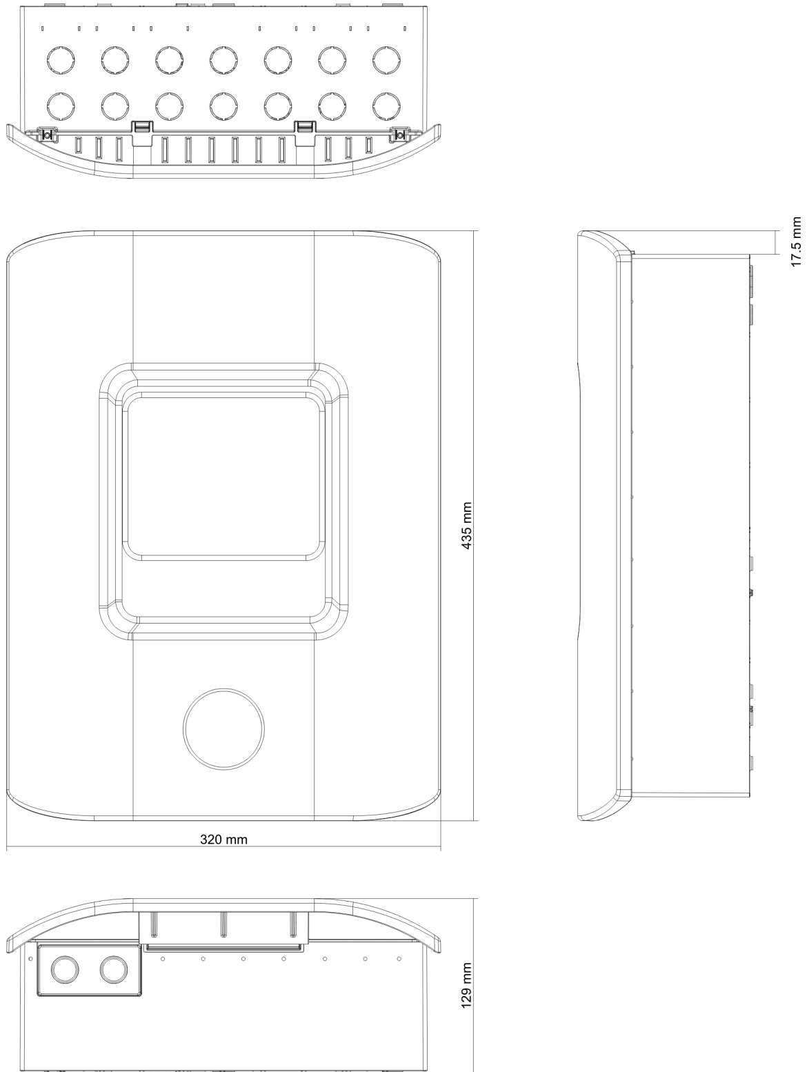
Afbeelding 21: Behuizing voor twee en vier groepen met deksel
