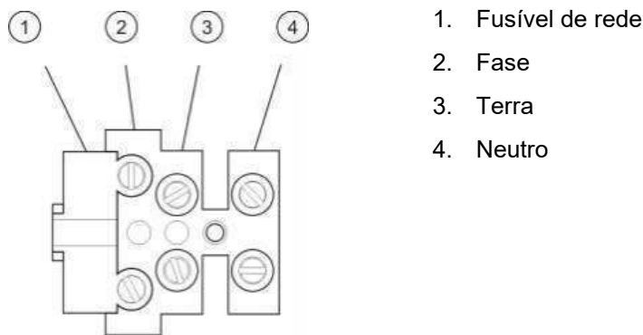
Figura 10: Ligação da alimentação de rede
