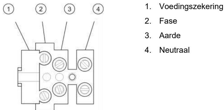
Afbeelding 10: De netvoeding aansluiten
