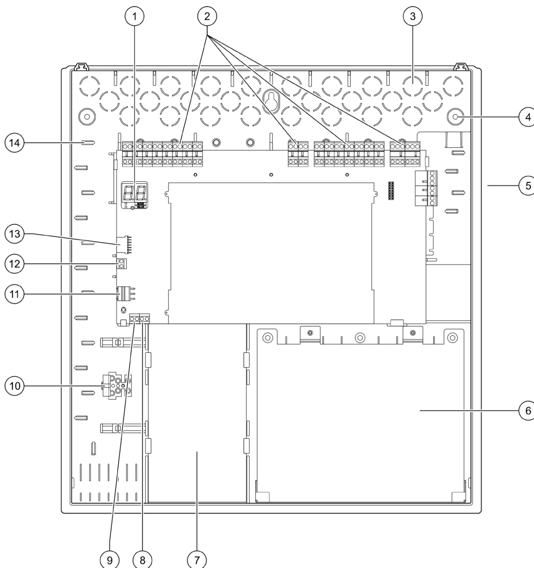
Afbeelding 2: Indeling behuizing voor acht-zone bedieningspanelen
