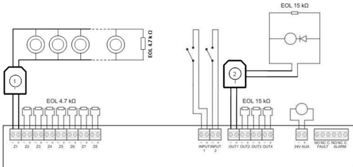
Afbeelding 7: Intrinsiek-veilige brandsysteemaansluitingen
