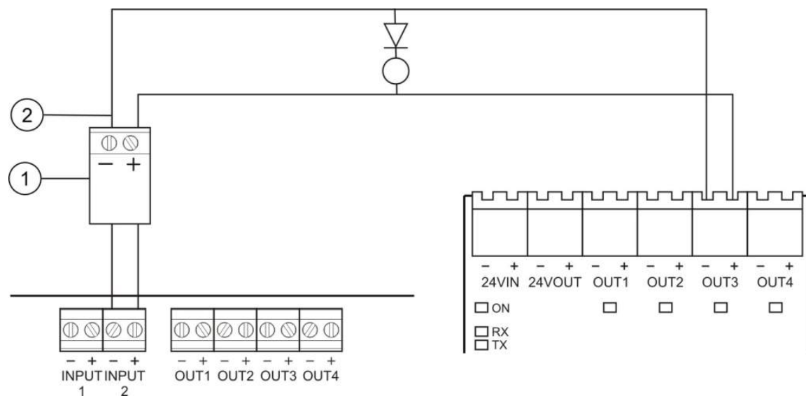
Afbeelding 9: Aansluiten op foutwaarschuwinguitgang
