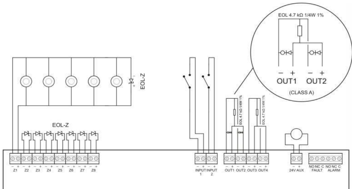
Afbeelding 5: EN 54-13 brandsysteemaansluitingen
