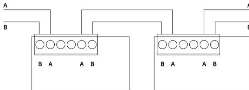
Afbeelding 13: Aansluitingen netwerkbord
