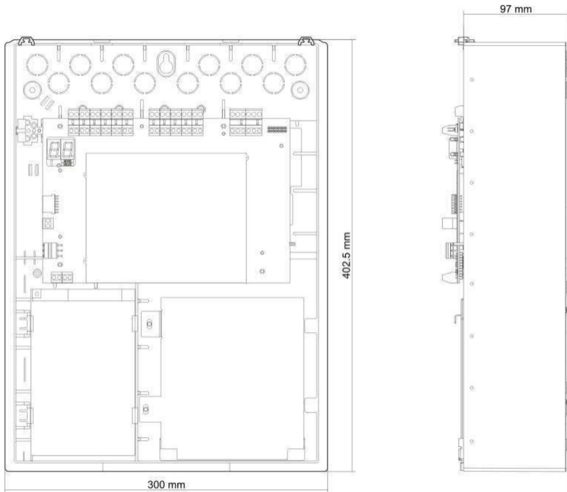
Bild 22: Två- och fyrasektioners skåp utan hölje
