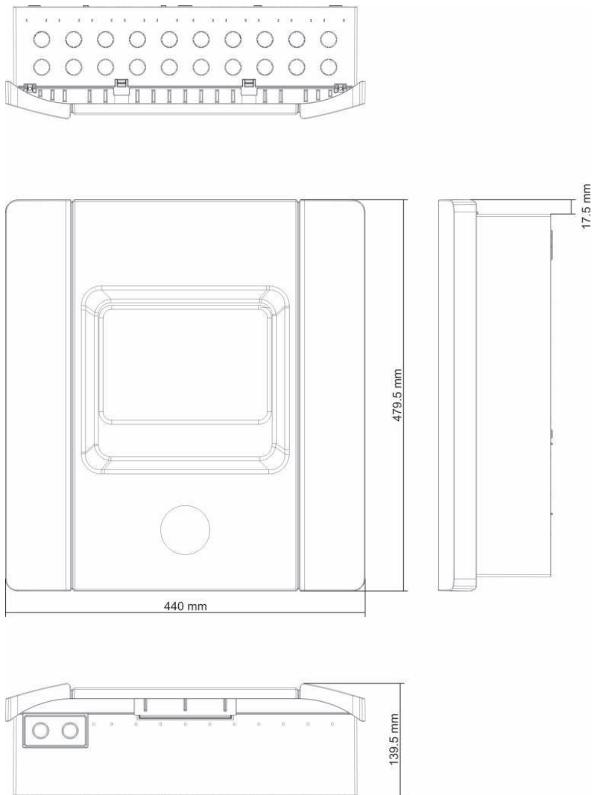
Bild 23: Åttasektioners skåp med hölje
