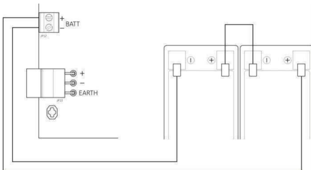
Bild 12: Ansluta batterierna
