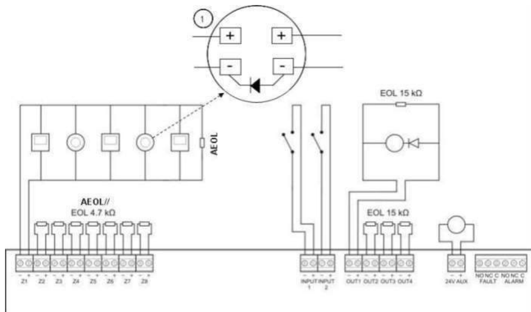
Bild 6: BS 5839-1 brandsystemanslutningar
