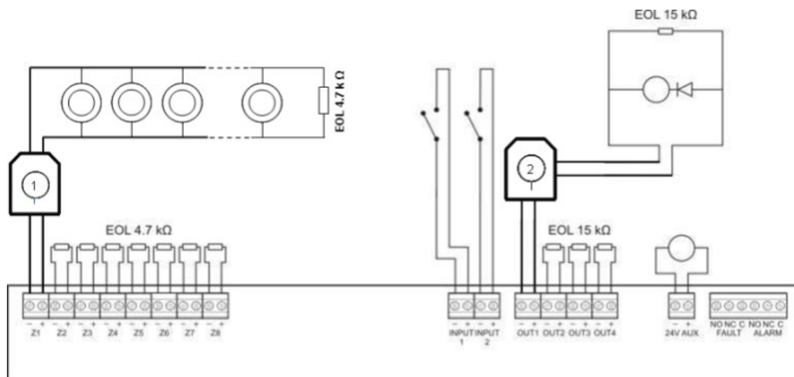
Bild 7: Egensäkra brandsystemanslutningar
