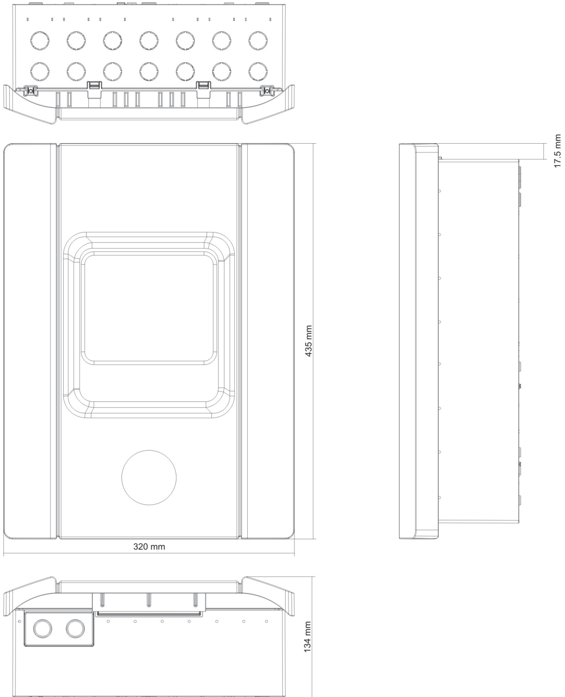
Figur 21: To- og firesoners kabinett med deksel
