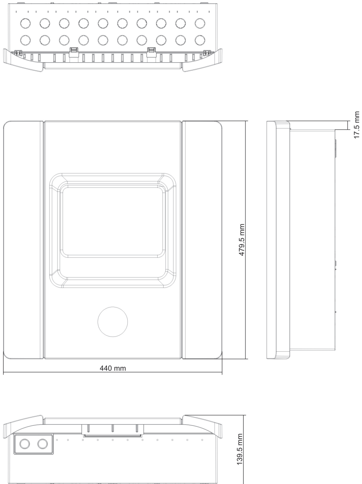
Figur 23: Åtte-soners kabinett med deksel
