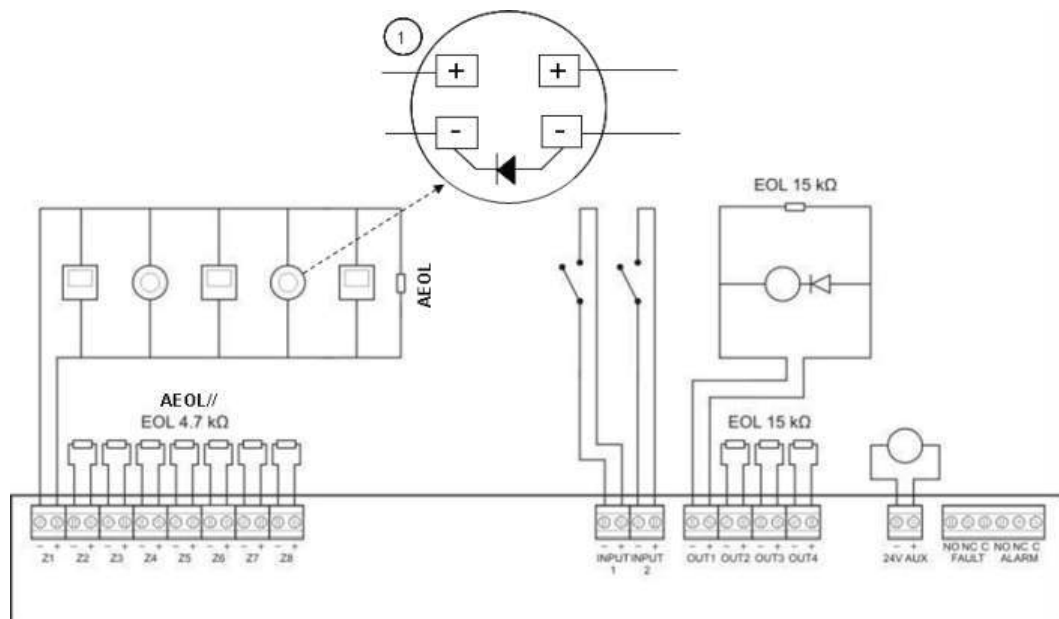
Figur 6: BS 5839-1-brannsystemforbindelser
