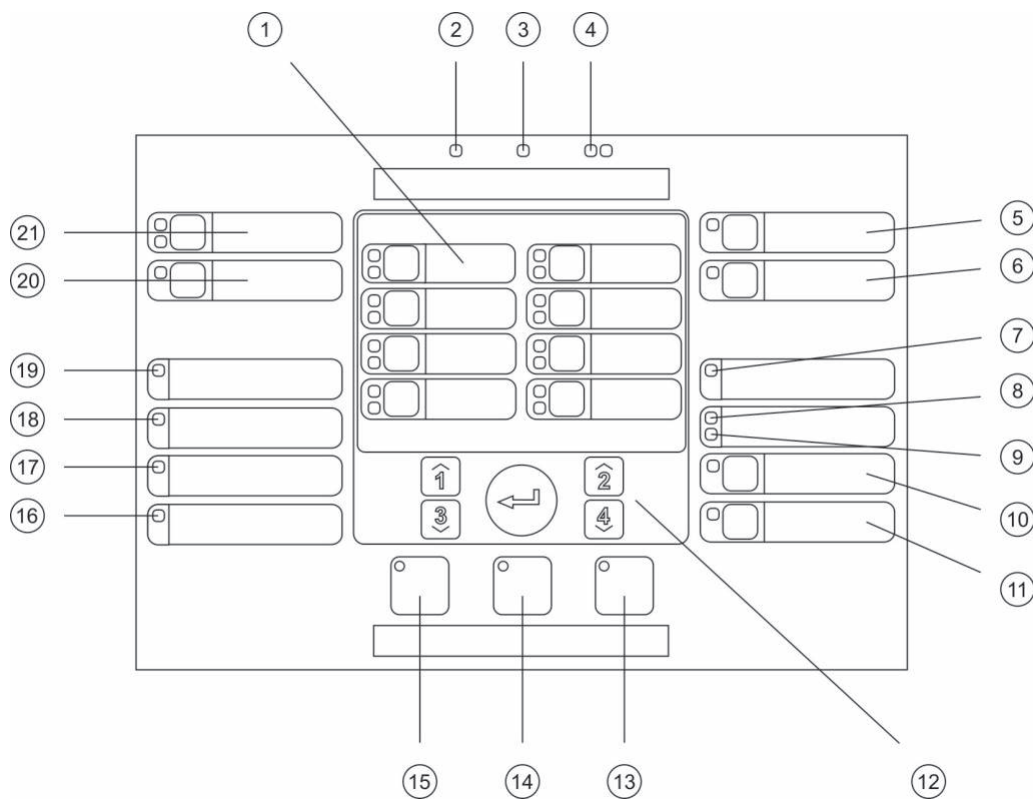
Figur 17: Brukergrensesnitt for sentraler med åtte soner
