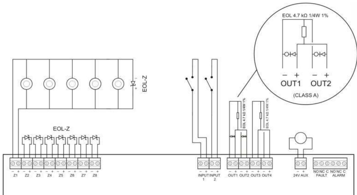
Figur 5: EN 54-13-brannsystemforbindelser
