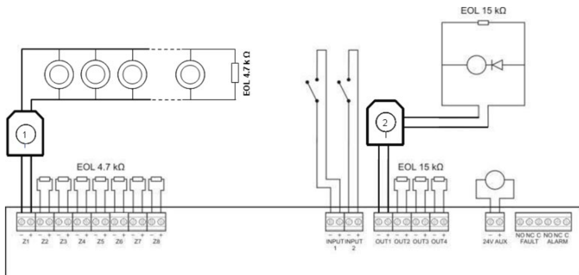
Figur 7: Eksplosjonssikre brannsystemforbindelser
