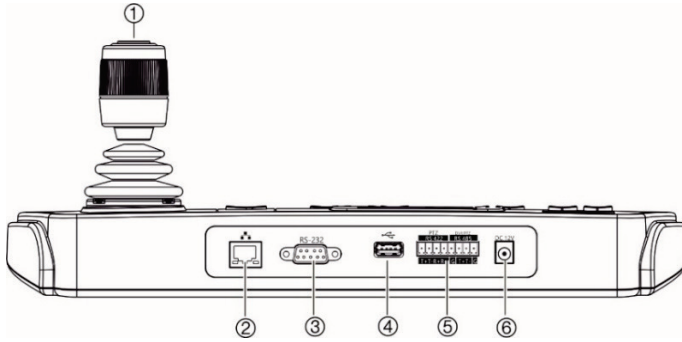
Şekil 1: Arka panel
