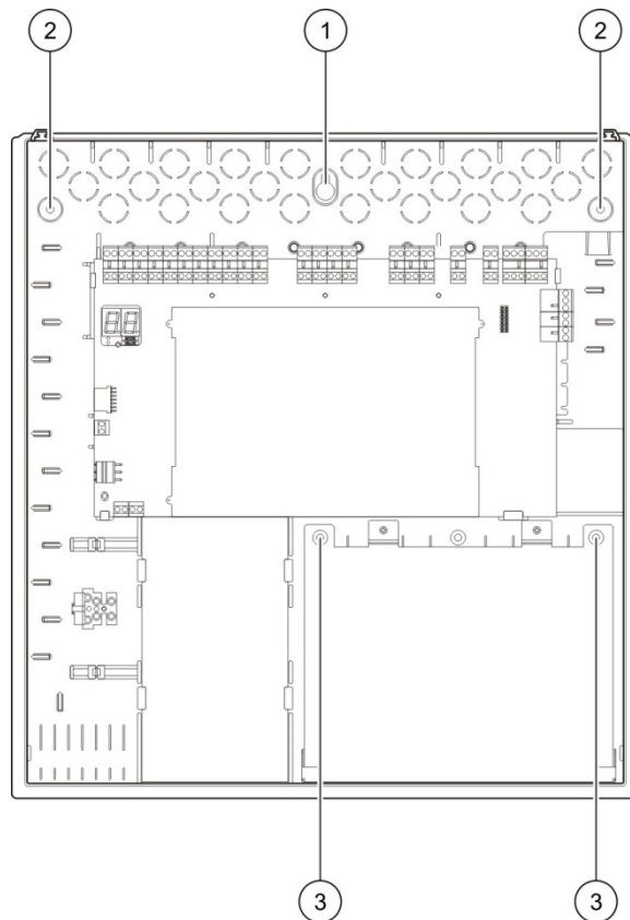
Figura 2: Posizioni dei fori di montaggio
