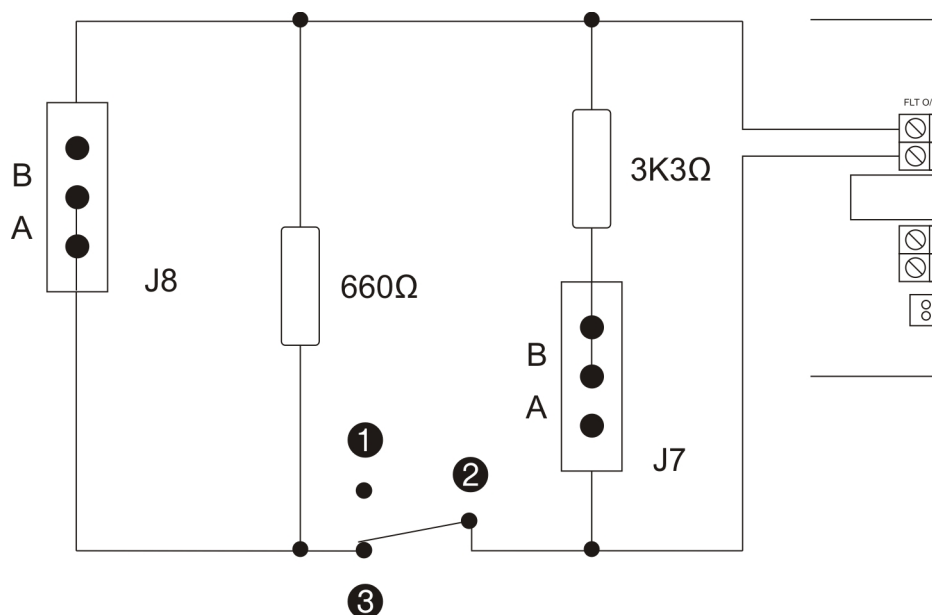
Afbeelding 19: Jumperconfiguraties van PS1200N-storingsrelais
