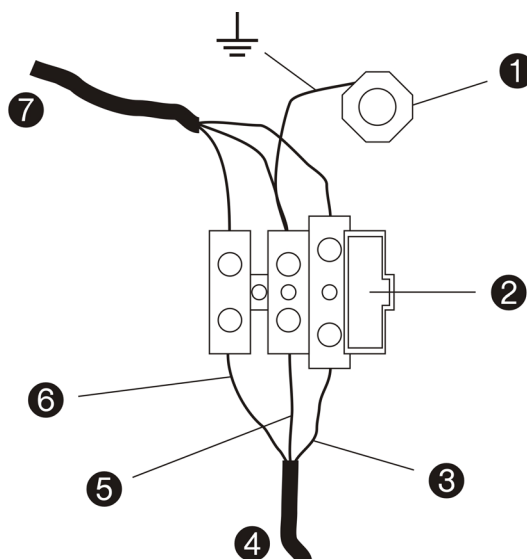
Afbeelding 17: Aansluitingen voor aansluitblok voor zekeringen
