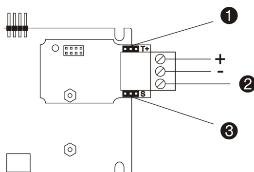
Afbeelding 12: NC2011-netwerkmodule
