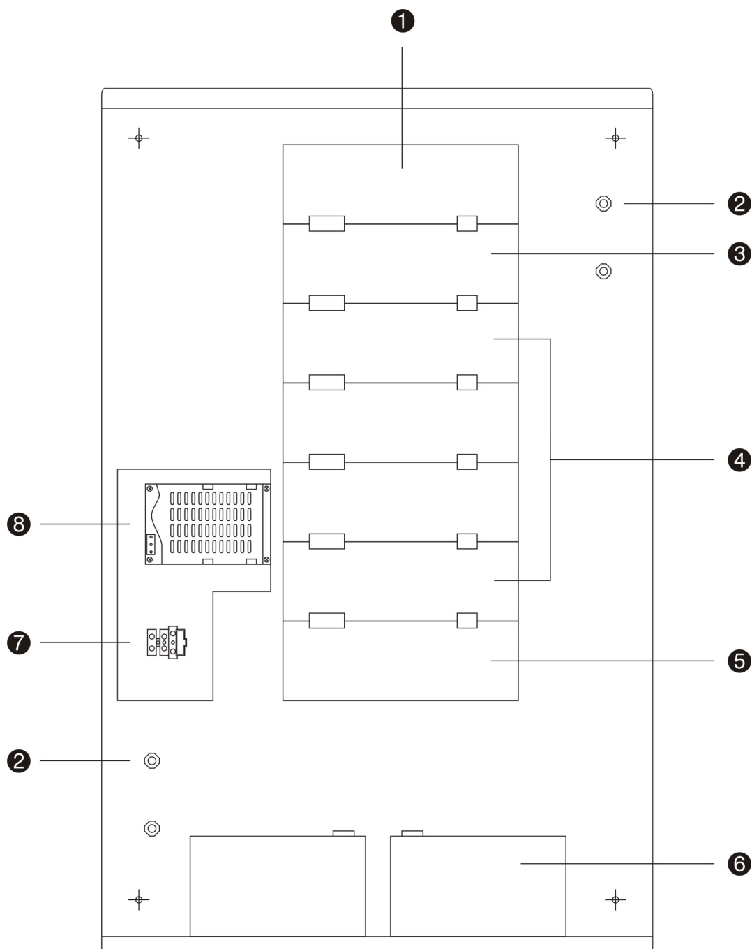
Afbeelding 2: Typische indeling van behuizing van 2000C-brandmeldpanelen
