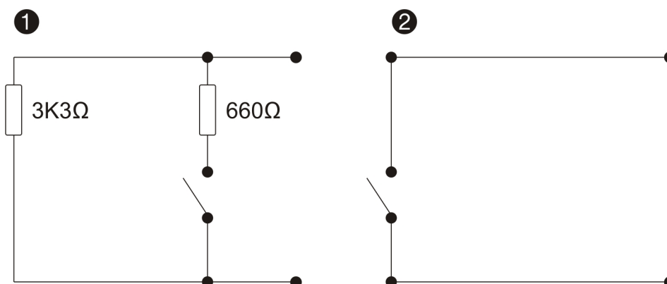
Afbeelding 8: Configuratieopties van jumpers
