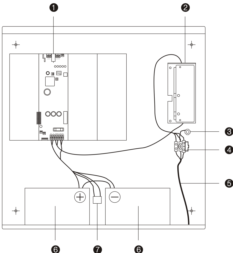
Afbeelding 15: Typische voedingsaansluitingen van een 1200C-brandmeldpaneel
