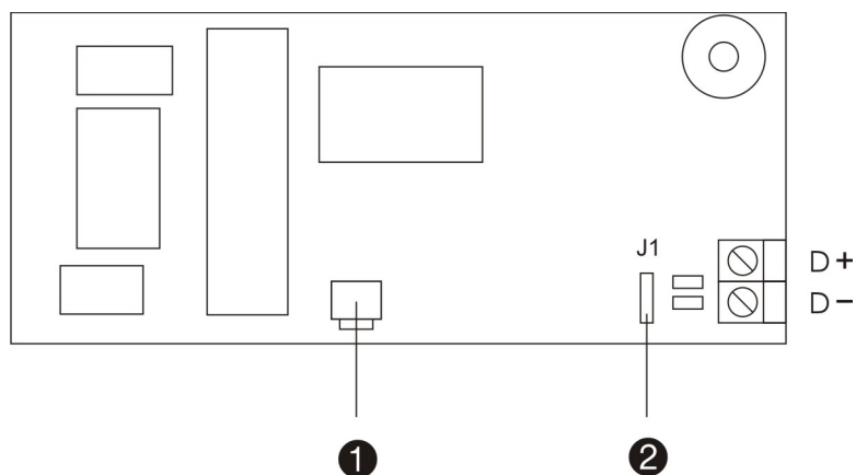
Afbeelding 14: LON2000-communicatiemodule
