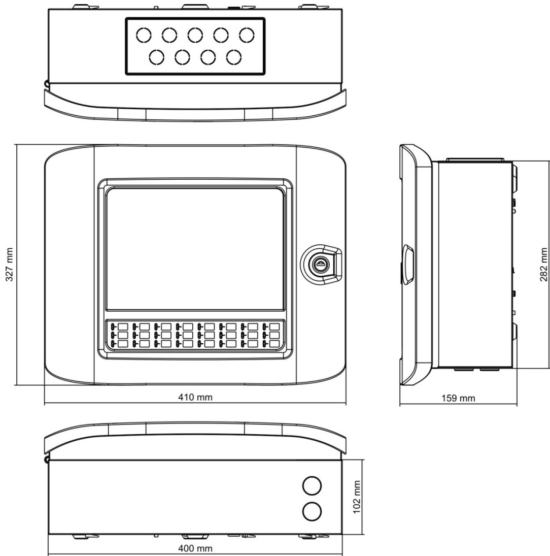
28 pav. Mažo korpuso matmenys ir vaizdai
