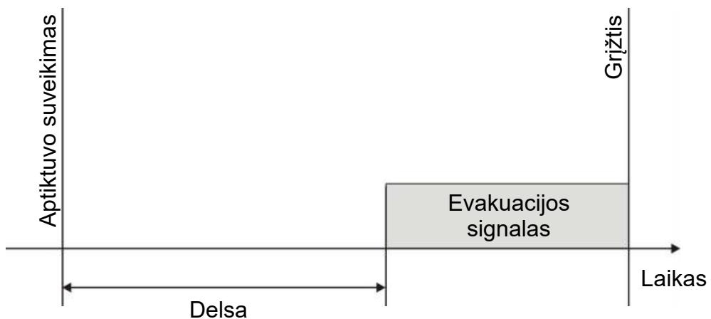
25 pav. Aptiktuvo suveikimas su standartine delsa (be antrojo etapo)
