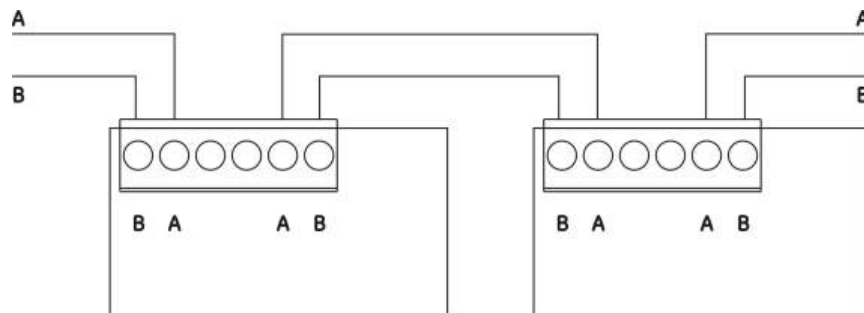
17 pav. Tinklo plokštės jungtys
