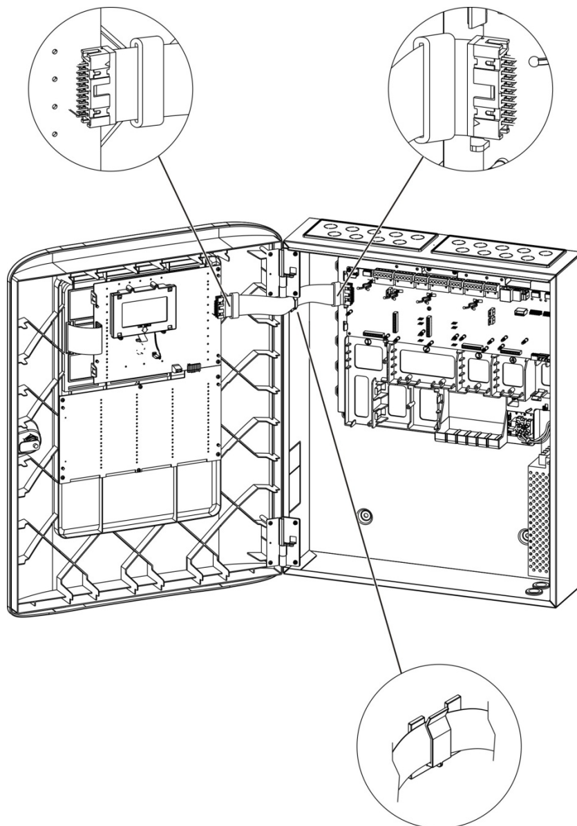
9 pav. Naudotojo sąsajos kabelio jungimas
