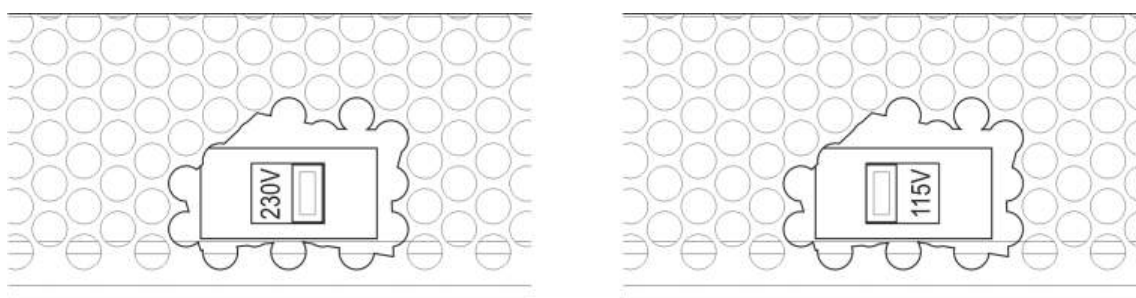
Figura 16: Selección de funcionamiento a 115 o 230 VCA
