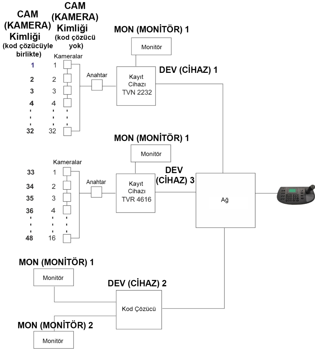
Şekil 15: Tuş takımı tarafından kontrol edilen bir sistem örneği
