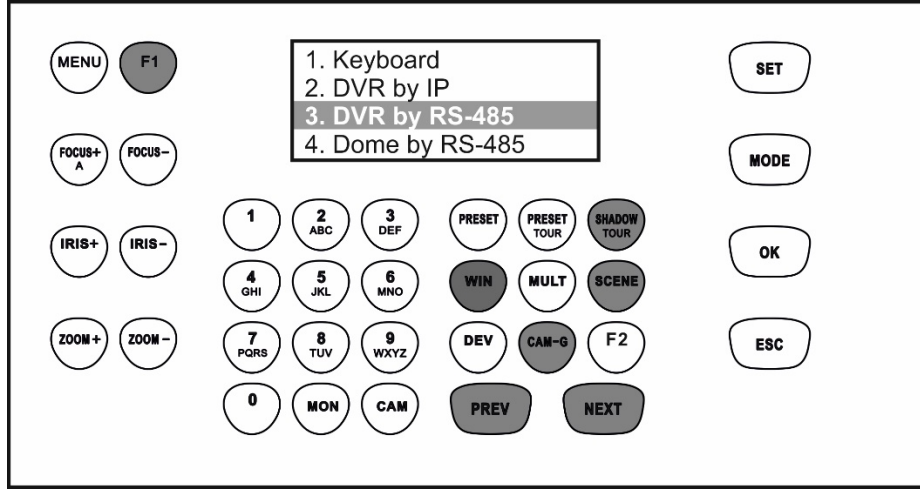
Şekil 21: DVR'yi RS-485 seri portunu kullanarak kontrol etme
