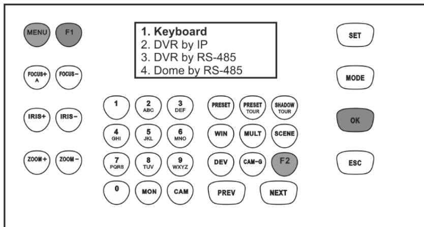
Şekil 19: Klavye modunda kullanılacak tuş takımı düğmeleri
