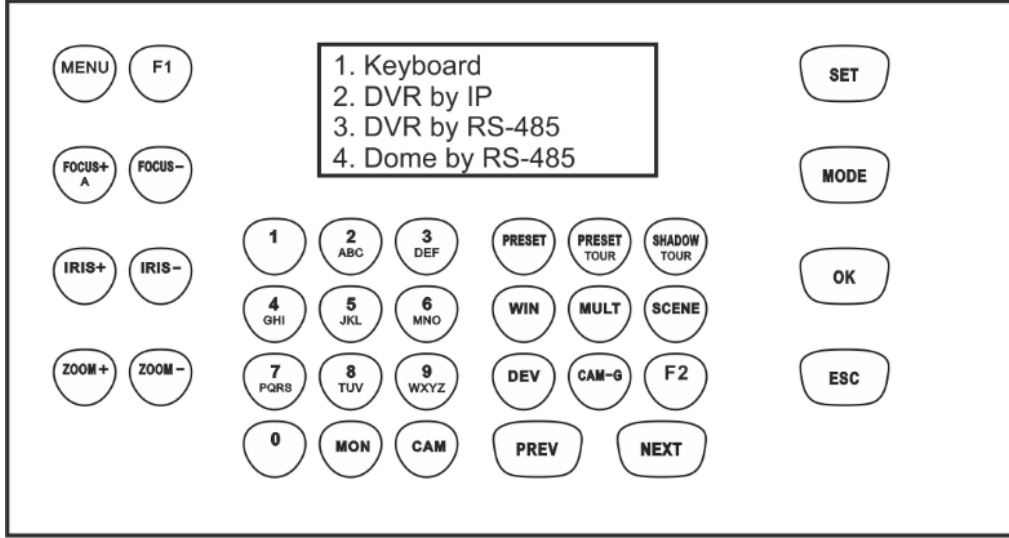
Şekil 2: Tuş takımı düğme yerleşimi
