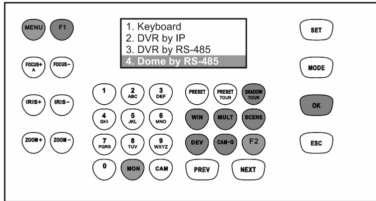
Şekil 22: Dome kameraları RS-485 seri portunu kullanarak kontrol etme
