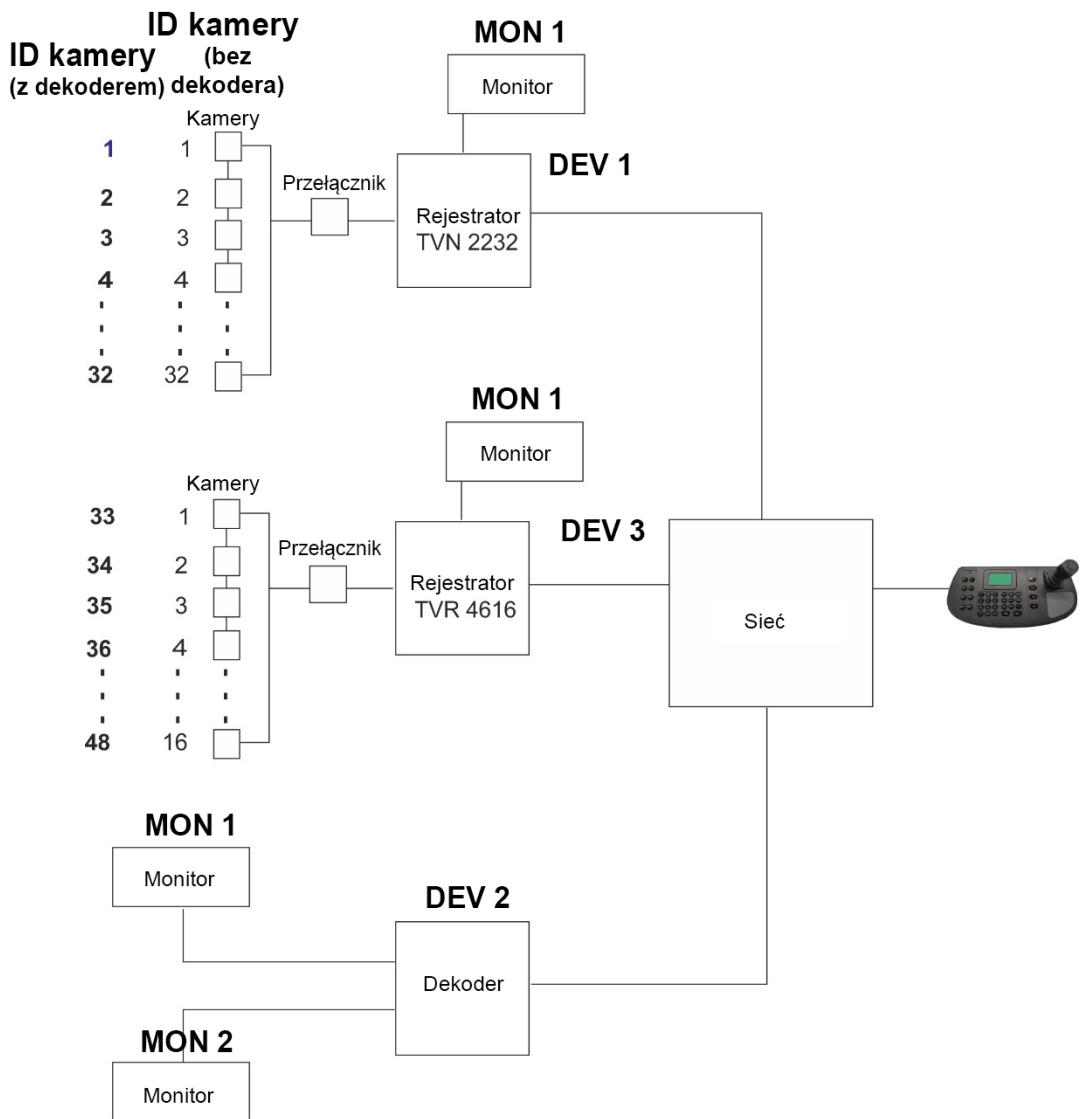
Rysunek 15: Przykładowy system sterowany za pomocą pulpitu
