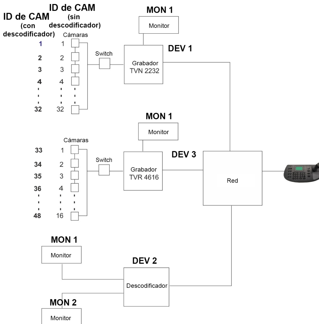
Figura 15: Ejemplo de un sistema controlado por un teclado
