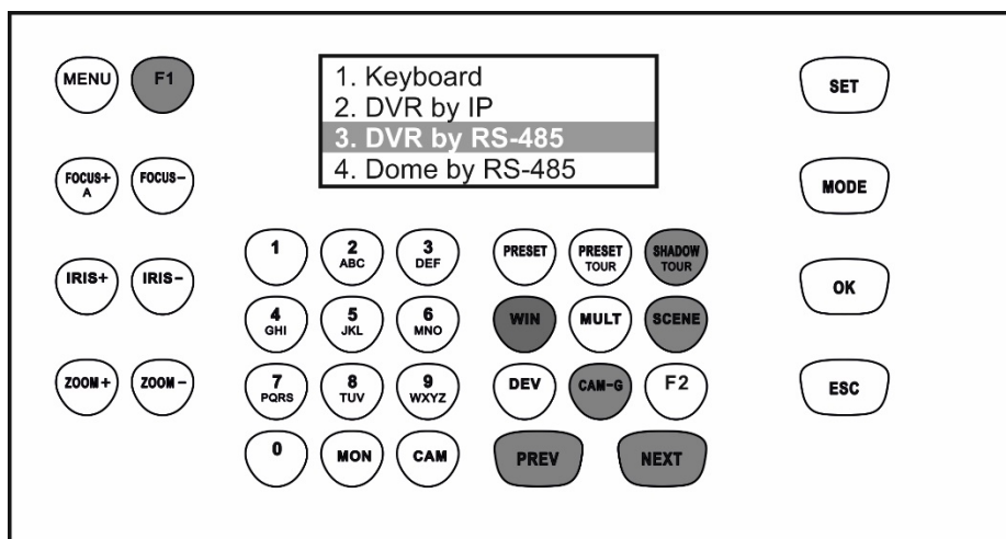
Figura 21: Control del DVR mediante el puerto serie RS-485
