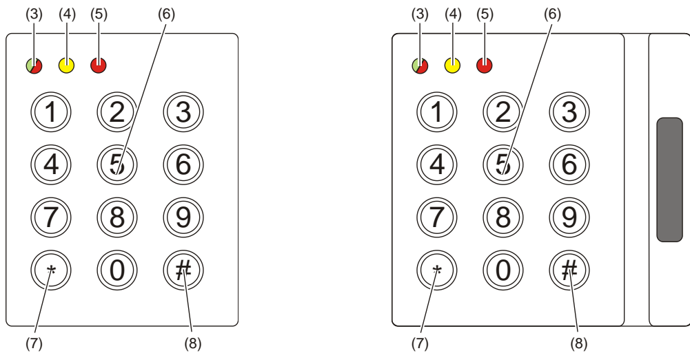
Kuva 5: ATS1151/ATS1156-lukijat
