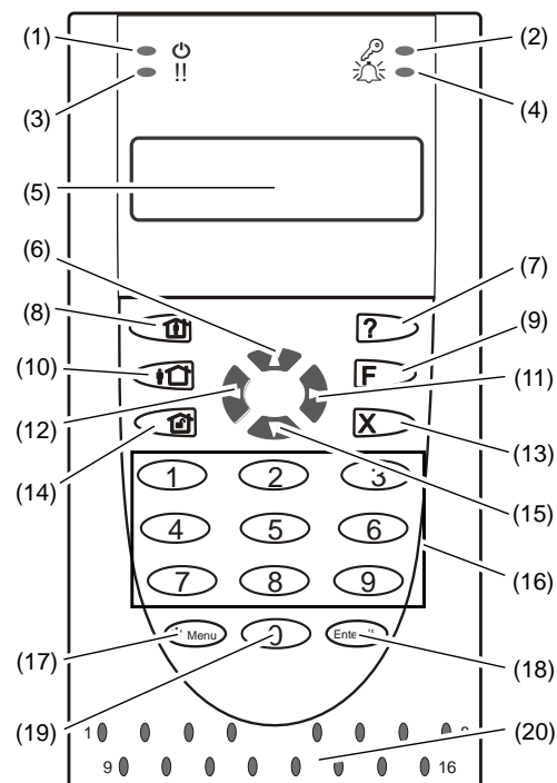
Kuva 1: ATS111xA-käyttölaite
