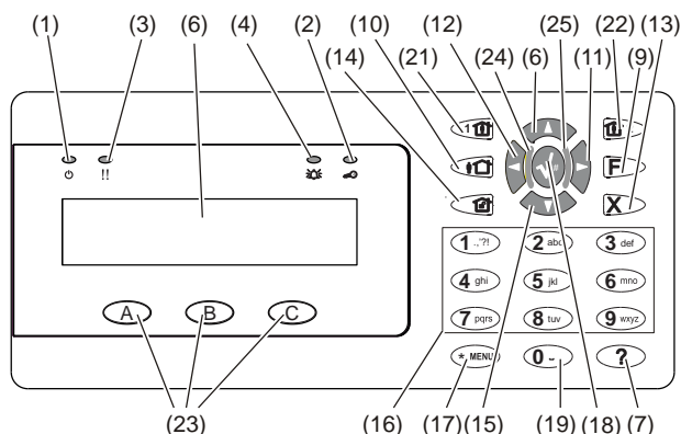
Figura 2: Tastiera ATS1135
