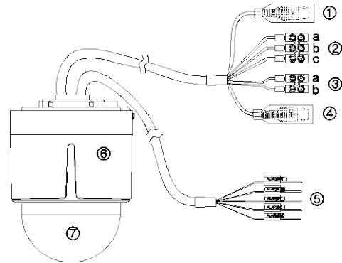
Rysunek 7: Wewnętrzna kamera kopułowa PTZ HD-TVI
