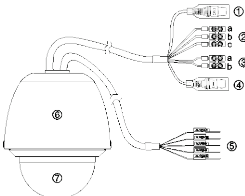
Rysunek 6: Zewnętrzna kamera kopułowa PTZ HD-TVI
