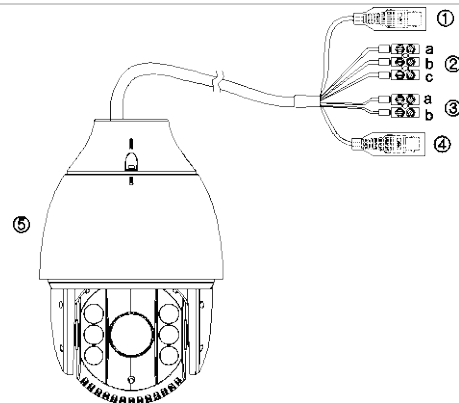
Rysunek 8: Zewnętrzna kamera kopułowa PTZ HD-TVI z podczerwienią
