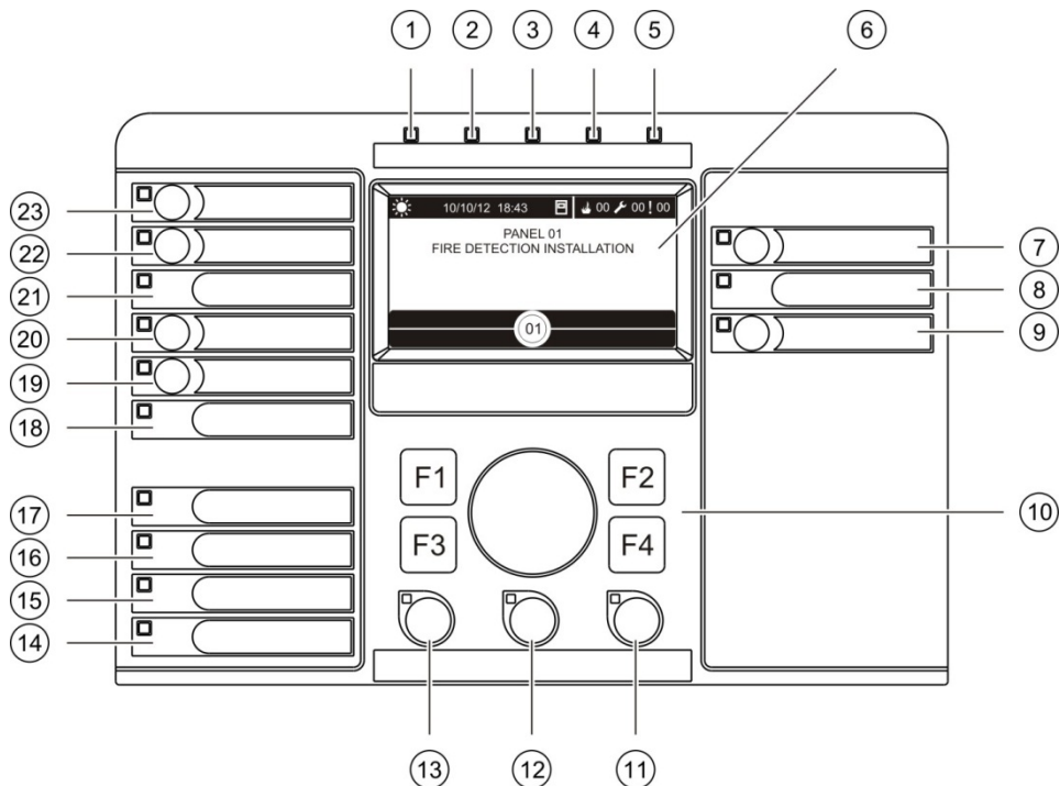
Kuva 1: Palohälyttilaitteen käyttöliittymä (sisältää paloreitityksen ja palontorjunnan ohjauksen)
