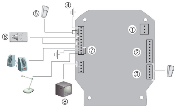
Figura 2: Connessioni al circuito stampato (esclusi i modelli TVP-1122/3122)
