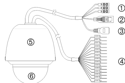
Figura 1: Panoramica della telecamera dome (viene mostrato montaggio a parete)
